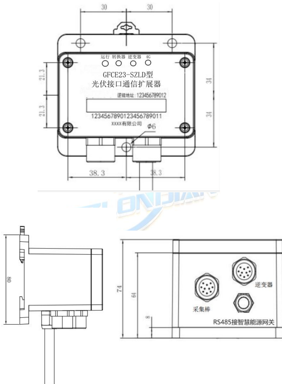
图 1-2 光伏接口通信扩展器外观结构图 01
