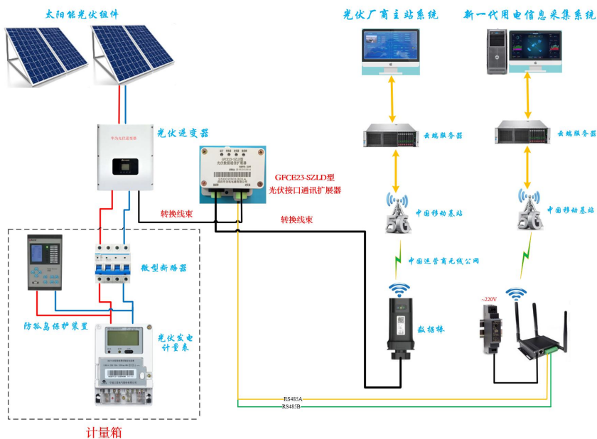
光伏接口通信扩展器网络架构拓扑图
