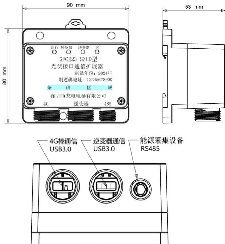
图 1-3 光伏接口通信扩展器外观结构图 02
